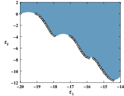
Fig. 3.7. NSGA-II on KUR.
